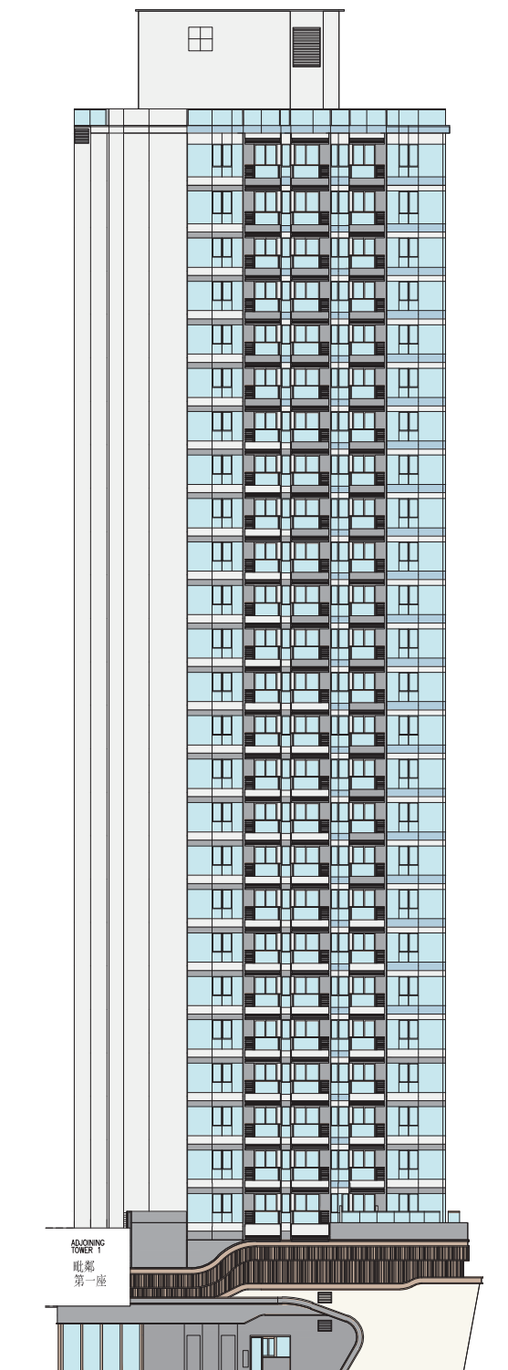
Elevation Plans 3 立面圖 3
