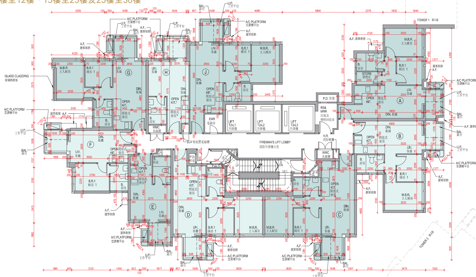
Tower 2 3/F, 5/F-12/F, 15/F-23/F & 25/F-30/F 第2座 3樓、5樓至12樓、15樓至23樓及25樓至30樓
